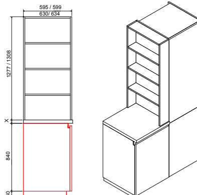
TERMINALE SOPRA TOP "MATRIX" PER BASI CON ZOCCOLO H 6 CON GOLA TERMINAL ABOVE WORKTOP "MATRIX" FOR BASE UNITS WITH PLINTH H 6 WITH FINGER RAIL
